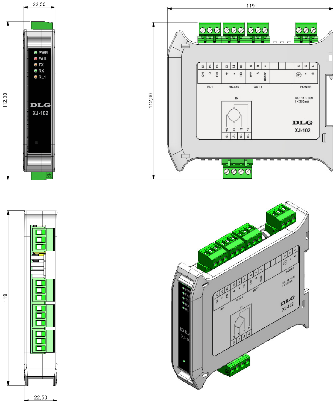
Figura 3 – Dimensionamento para montagem (Cotas em milímetros)
