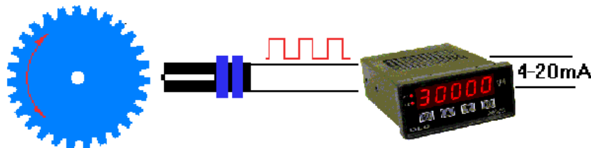
Figura 3 - Uso do pick-up com indicador IM-110
